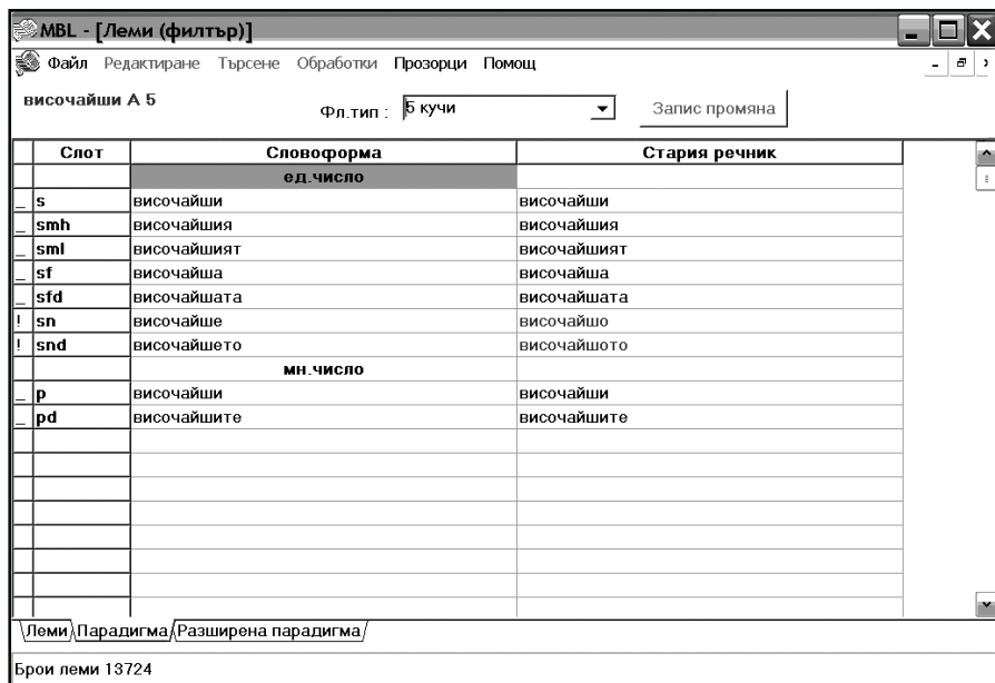
Фиг. 2. Сравнение между две версии на речника – текуща и минала – за определена лема в процеса на генериране на нейните форми, със сигнализация за различаващи се словоформи в двете версии.
